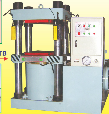
四柱上移式油压机
